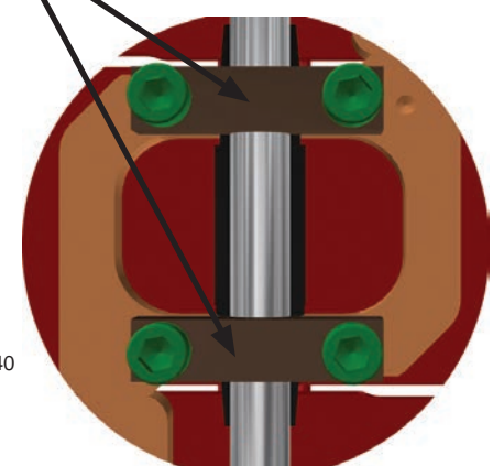
Détail A Étape n° 4
