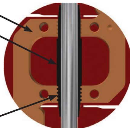
Détail A Étape n° 3
